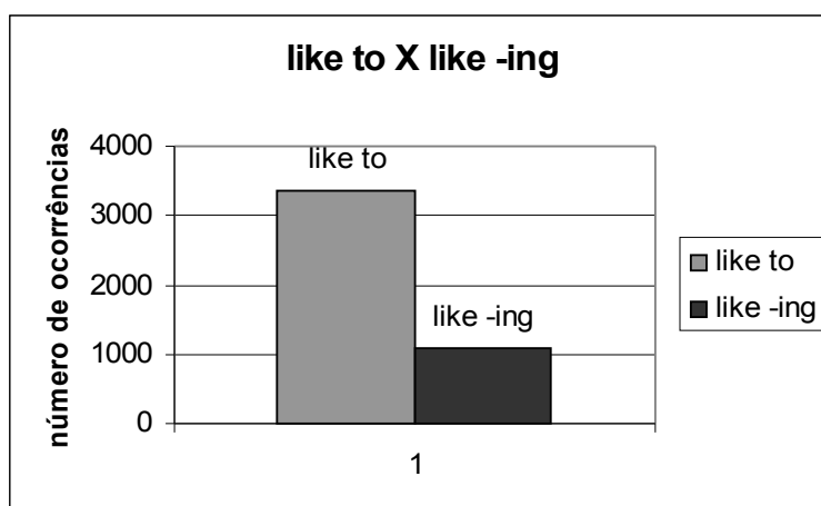
Gráfico 1- Probabilidade de ocorrência de infinitivo e gerúndio com like
