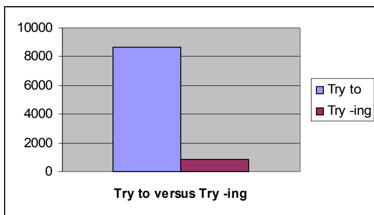
Gráfico 3- Frequência de ocorrência de infinitivo e gerúndio com try
