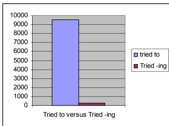
Gráfico 5- Freqüência de ocorrência de infinitivo e gerúndio com tried
