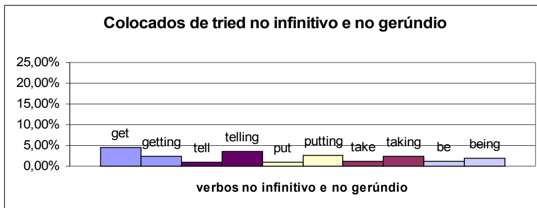
Gráfico 6- Freqüência dos cinco primeiros colocados de tried no infinitivo ou no gerúndio.
